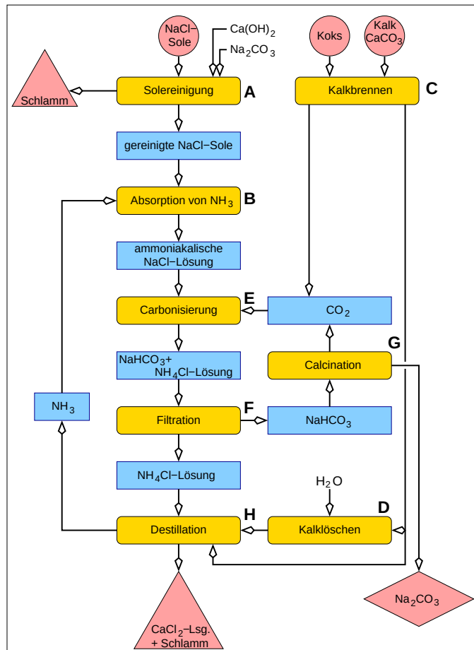
Prozess-Schema Solvay-Verfahren
