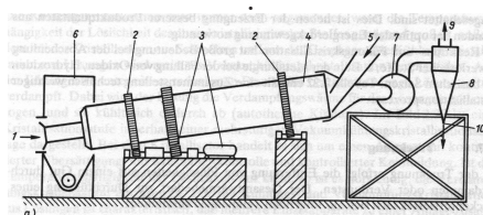
Drehrohrföfen G
