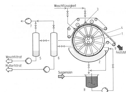
Vakuumdrehfilter F
