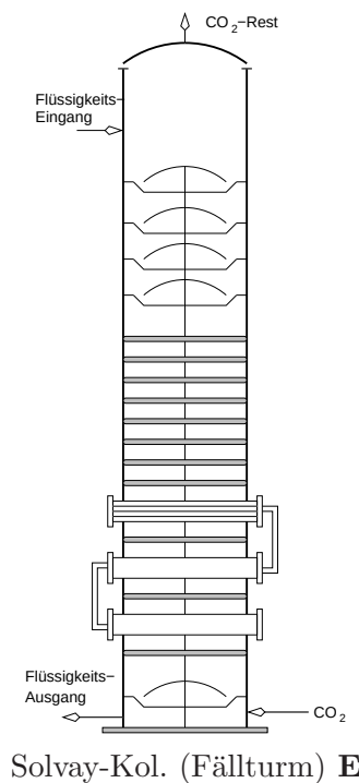
Prozess-Schema Solvay-Verfahren
