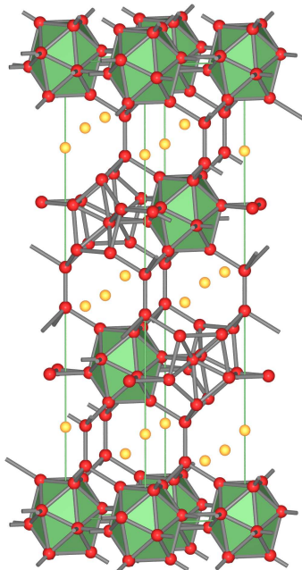
\text{RbGa}_7
