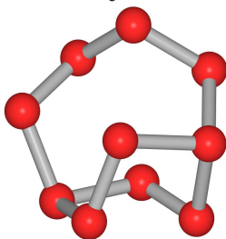
\text{Se}_{10}^{2+}
