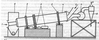
Drehrohrföfen
