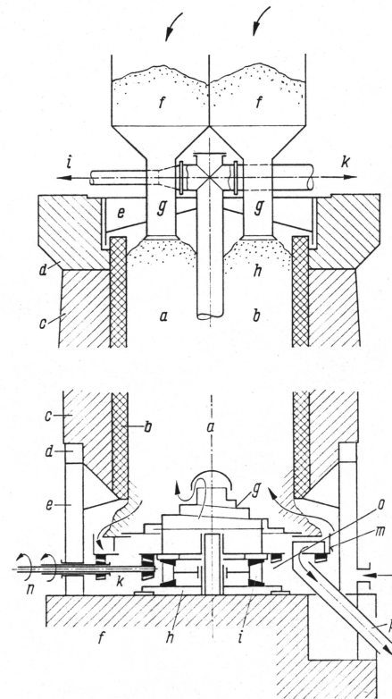
Kalkofen
