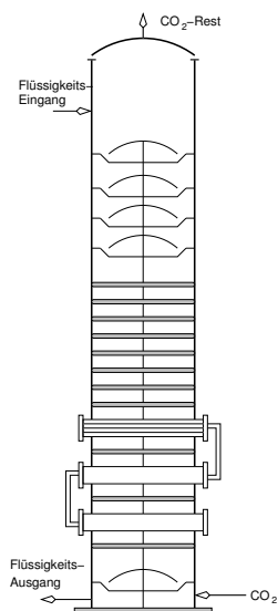
Solvay-Kolonne (Fällturm)
