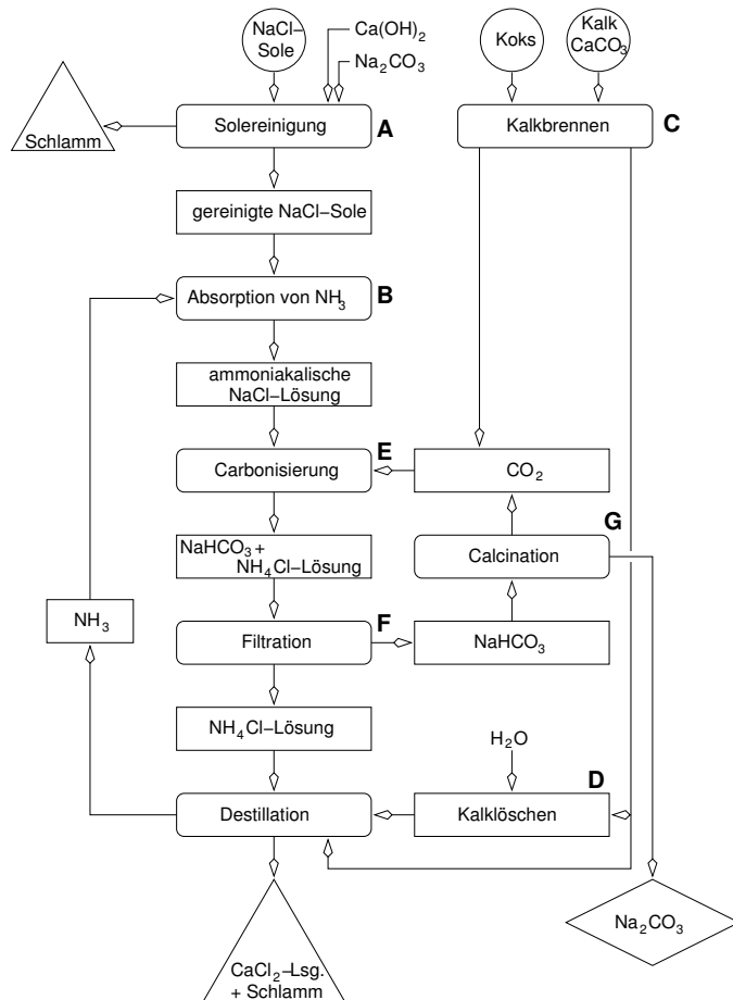
Prozess-Schema Solvay-Verfahren
