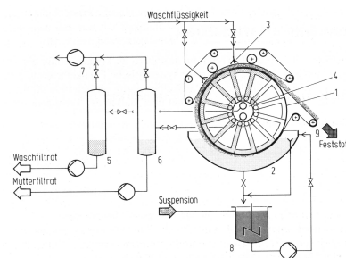
Vakuumdrehfilter
