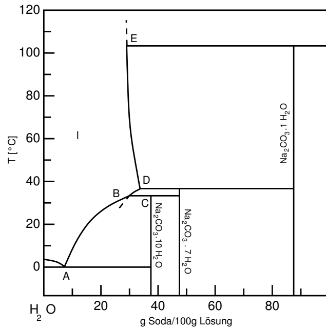
Phasendiagramm \text{Na}_2\text{CO}_3 - \text{H}_2\text{O}
