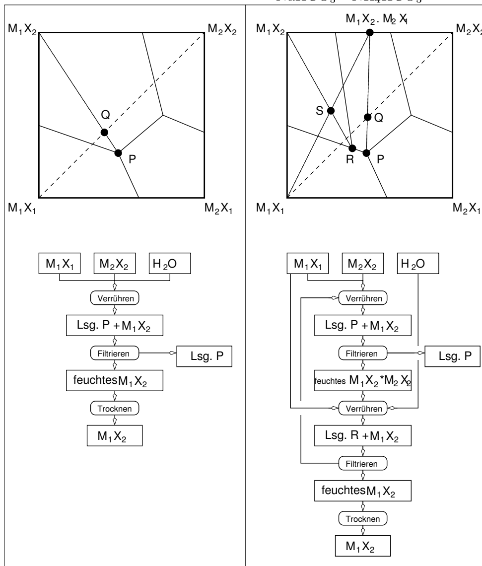
Gleichgewichtsdiagramme reziproker Umsetzungen (nach Jänecke)
