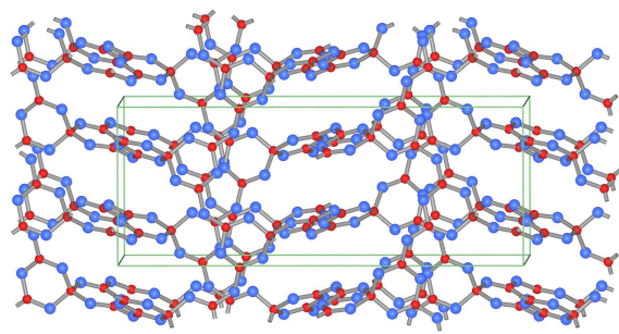
KB_5O_8
