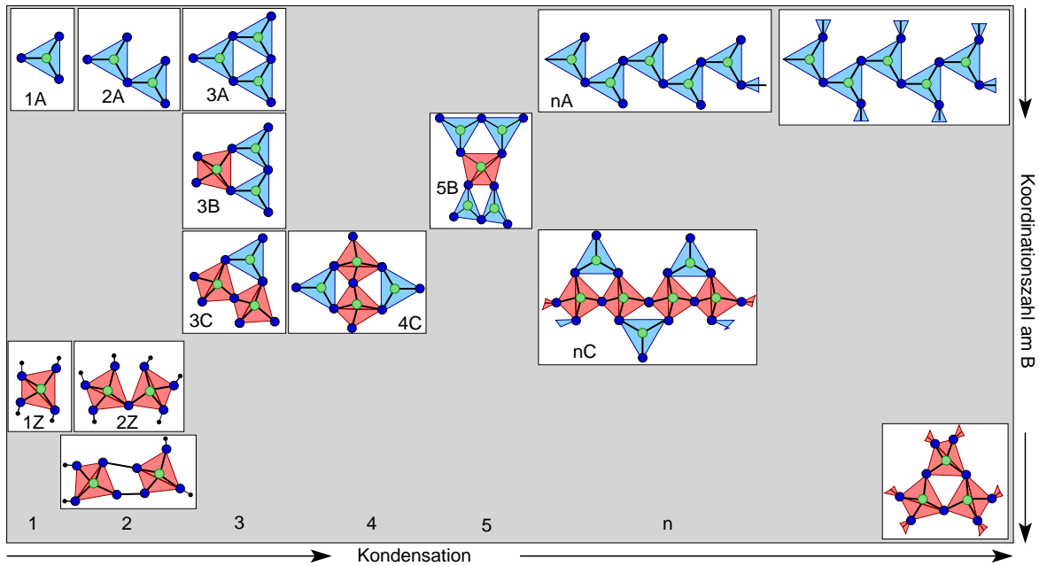
\alpha - B_2O_3
