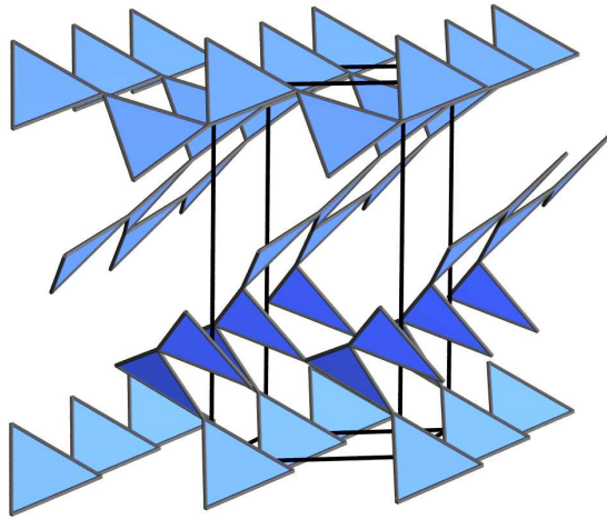
\alpha - B_2O_3
