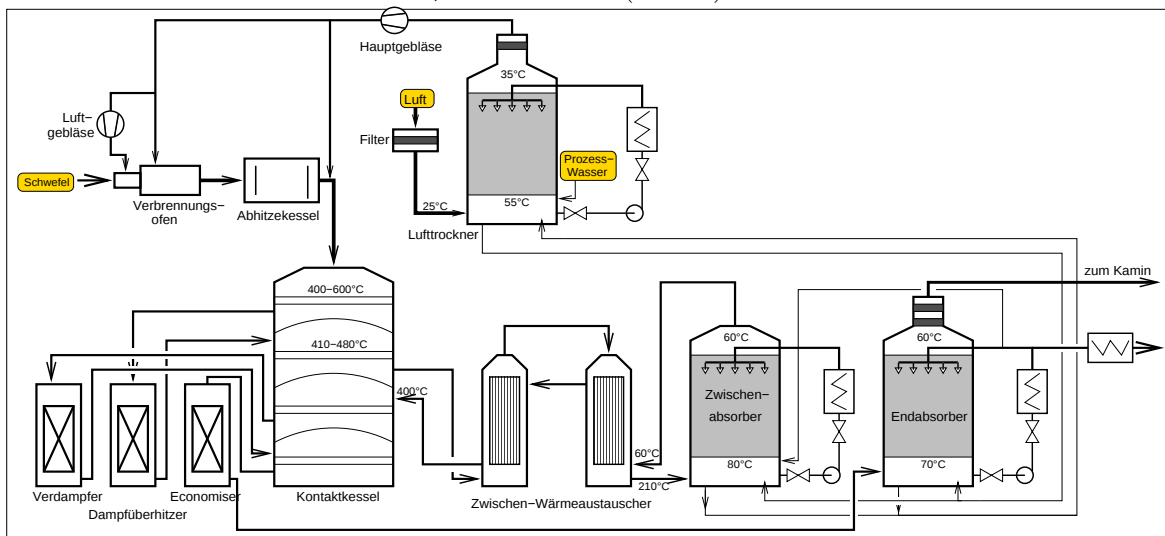
Schwefelsäure-Doppelkontaktverfahren: Anlagenschema
