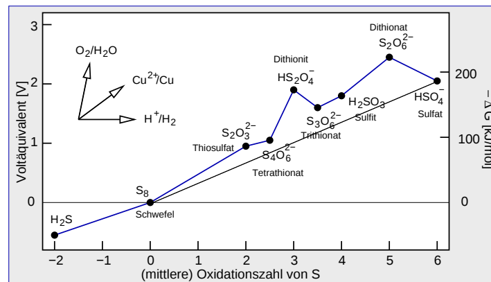
Voltäquivalentdiagramm verschiedener S-Spezies in saurer Lösung
