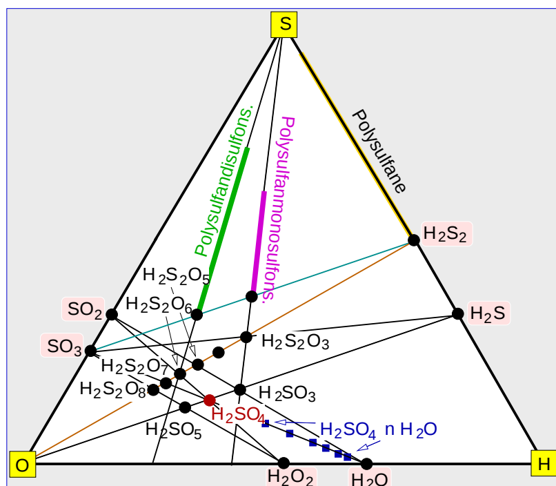
Sauerstoffsäuren des Schwefels im Lagediagramm S-O-H
