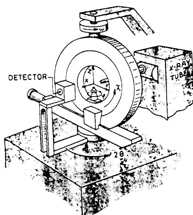
Vierkreisdiffraktometer
