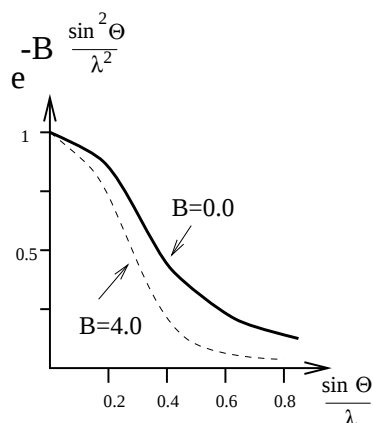
Temperaturfaktoren
