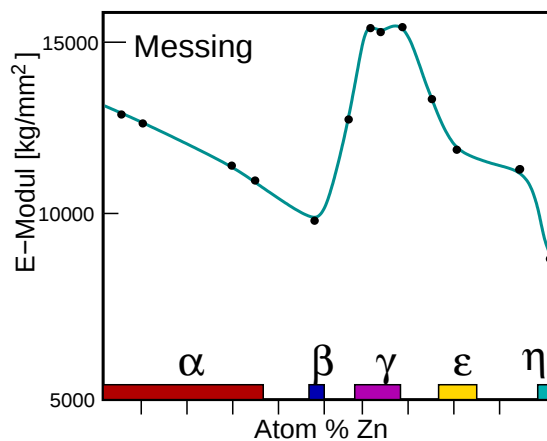
Mechanische Eigenschaften von Messing (links) und Bronze (rechts)
