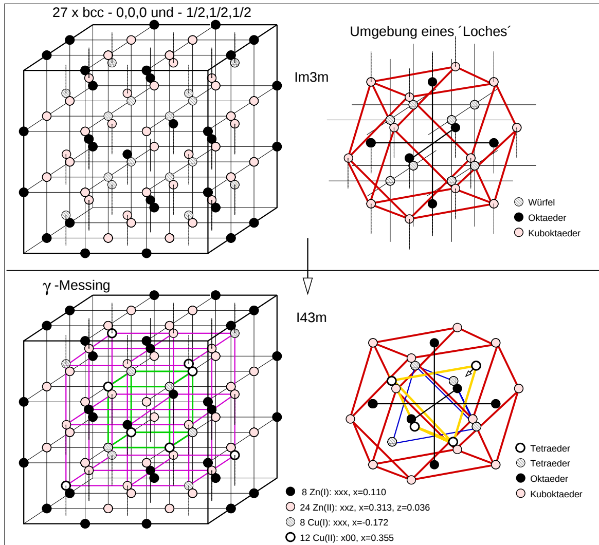
Struktur von γ-Messing
