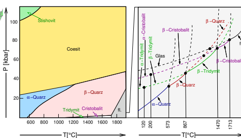
p-T-Diagramm
