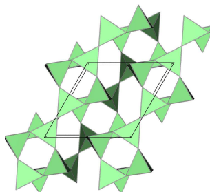
Coesit
