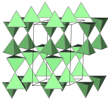
Tridymit
