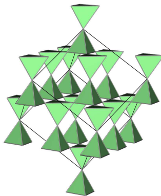
Cristobalit
