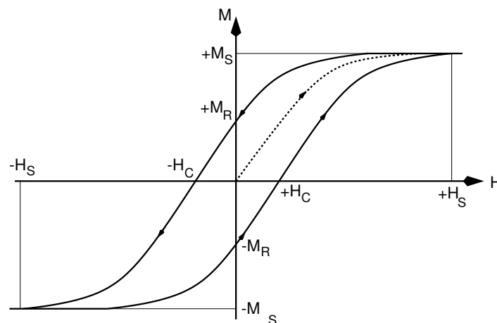
Hysteresis bei Ferro- und Ferrimagnetika
