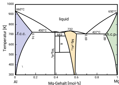
Phasendiagramm Al-Mg
