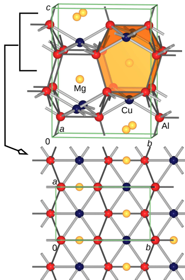
Kristallstruktur der S-Phase \text{MgCuAl}_2
