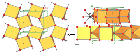
Struktur von \text{Fe}_3\text{C} (s. 9. Stunde)
