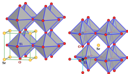
2 \times Perowskit-Struktur
