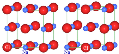
2 \times Kochsalz-Struktur
