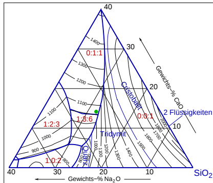
Phasendiagramm \text{Na}_2\text{O}-\text{CaO}-\text{SiO}_2
