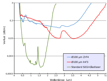
Verluste bei \text{ZrF}_4 -, \text{InF}_3 - und \text{SiO}_2 -basierten Glasfasern
